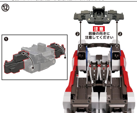
⑪SRX用太ももカバーを図の位置に取り付けます。⑫①両翼基部の左右を図のように動かします。②両翼基部の前後の向きに注意して図の位置に取り付けます。
